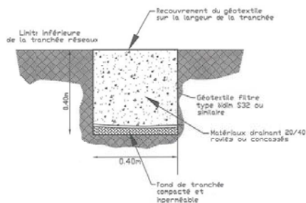
Schéma type de drain
